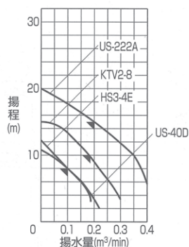
■性能曲線
