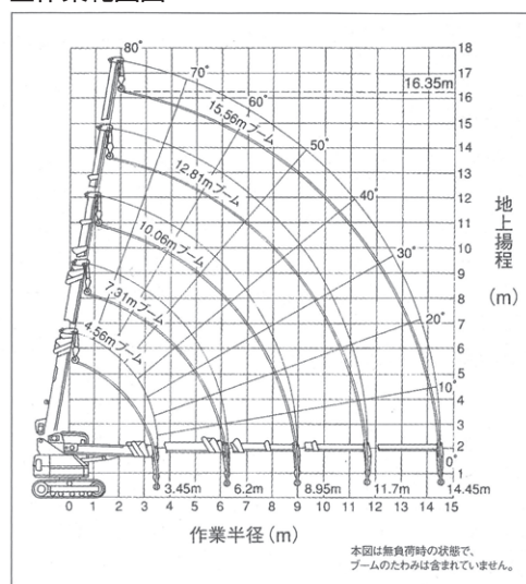
■作業範囲図
