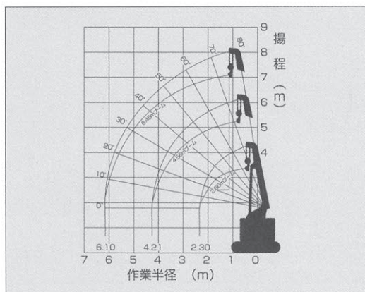
■作業範囲図
