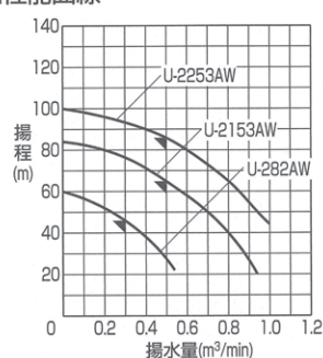
■性能曲線
