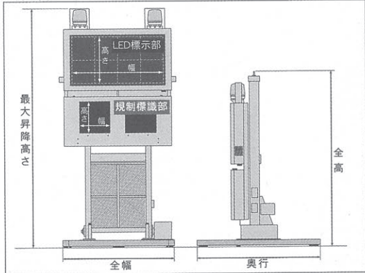
■外形図
