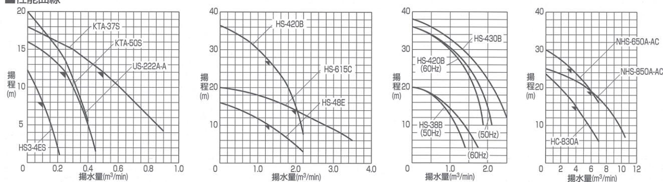
■性能曲線
